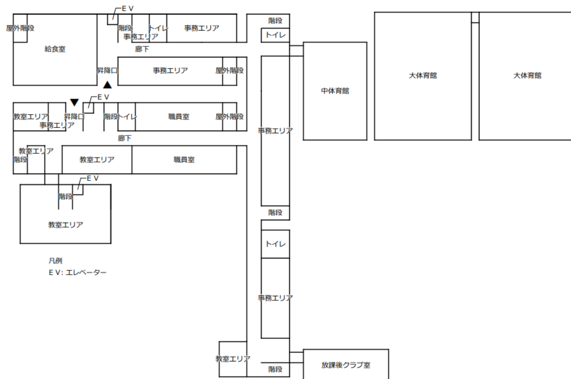
【1階平面図】
