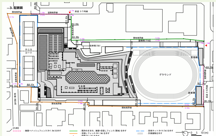
配置図
